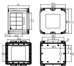
JBX884 - JBX887
