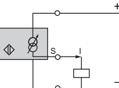
Branchement "3 fils"
